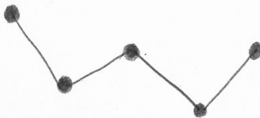
Cariopea
